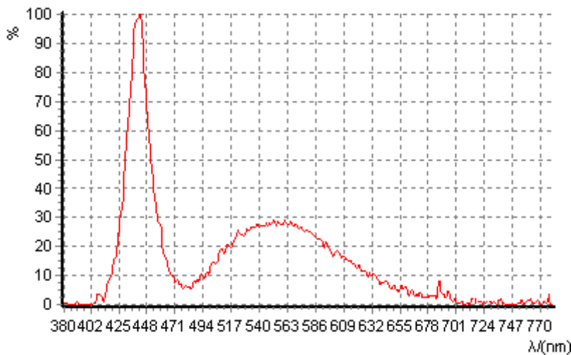
相对光谱分布曲线 Relative Spectral Distribution Curve
